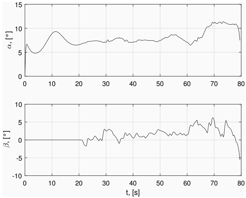
Slika 7.11: Napadni kut i kut klizanja letjelice
