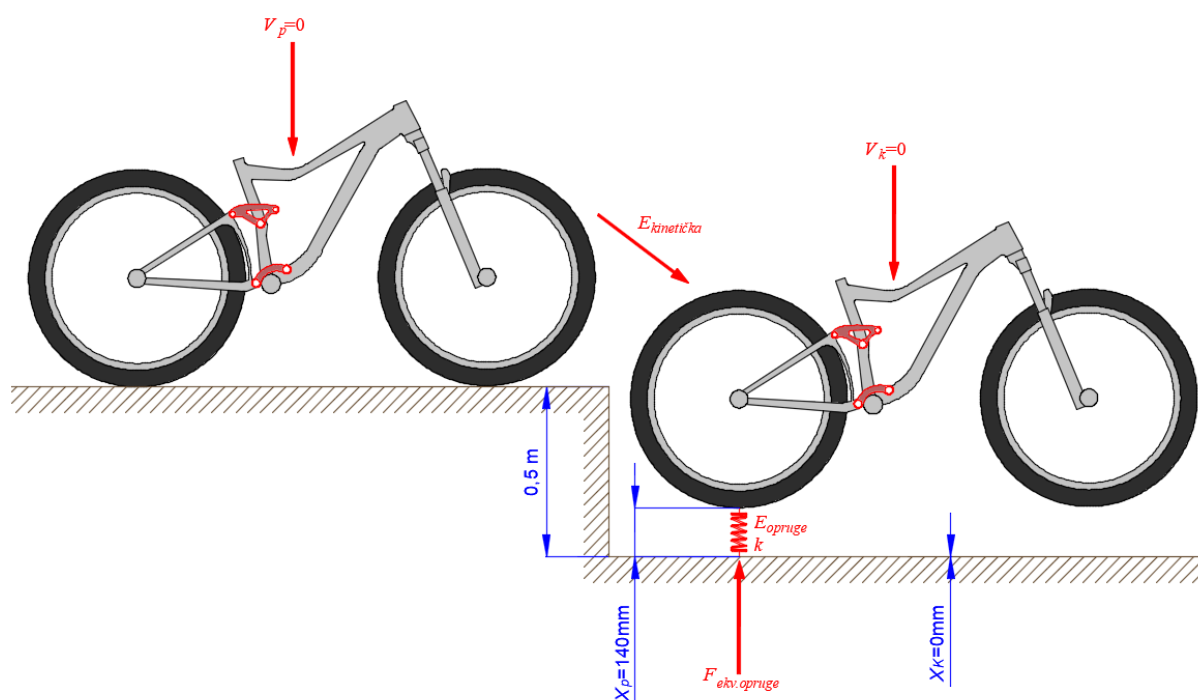
Slika 24. Proračunska skica promatranog bicikla
