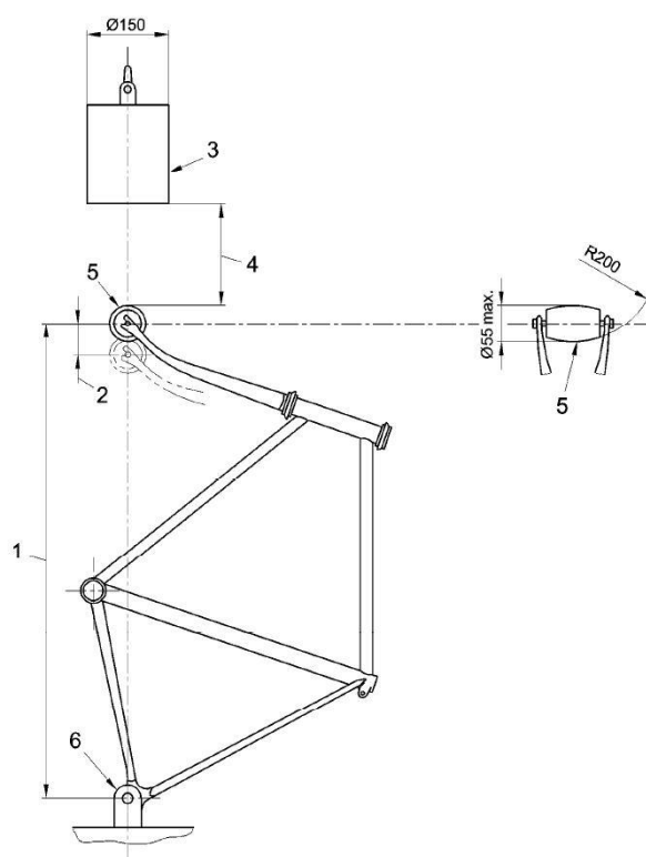
Slika 8. Ispitivanje okvira padajućim utegom [10]
