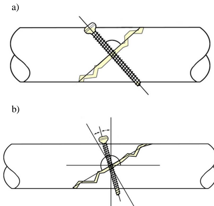
Slika 15. Kompresija ostvarena vijkom: a) pravilno i b) nepravilno postavljene vijak [21]
