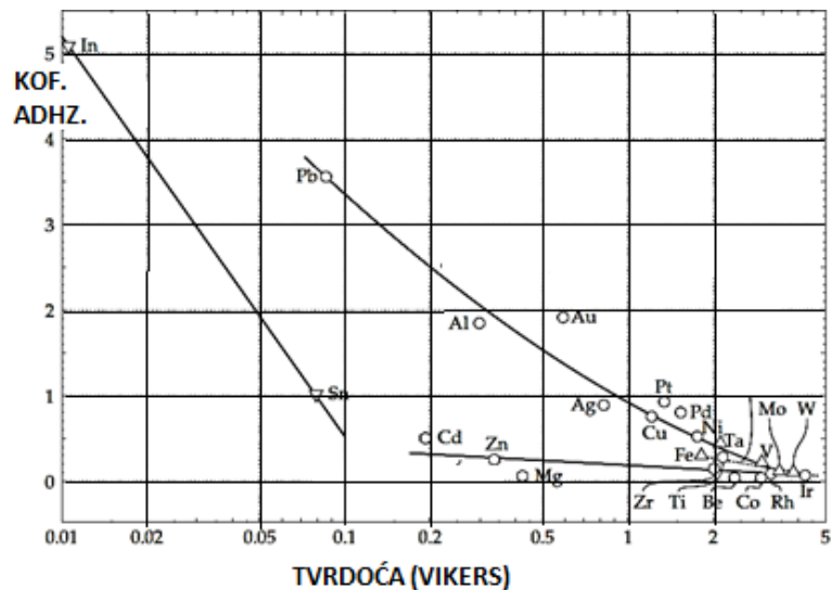
Slika 5.7. Otvrdnuće zbog mehanizama uslijed trenja [12]
