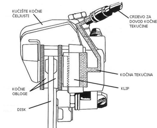
Slika 4.2. Mehанизam djelovanja kočione čeljusti [2]
