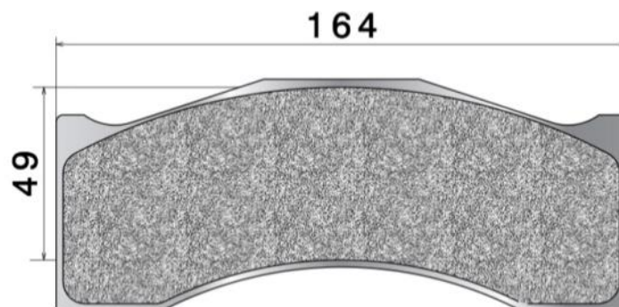
Slika 6.1 Dimenzije kočione obloge
