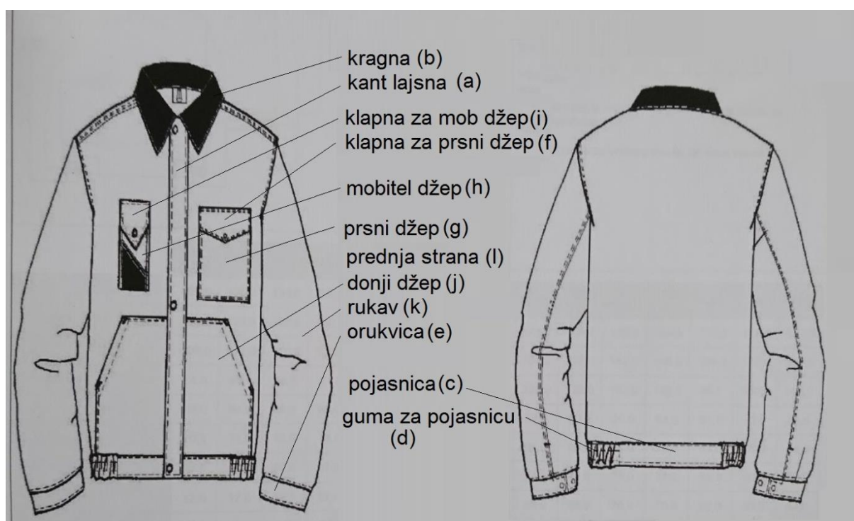
Slika 9. Skica proizvoda
