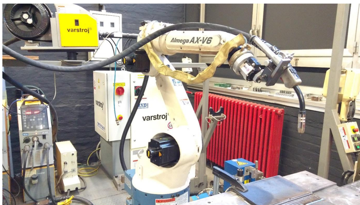
Slika 38. Robotska stanica Almega OTC AX V6
