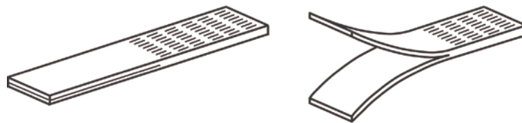
Slika 27 Skica uzorka sa prethodnim uzdužnim šivanjem slojeva [2]
