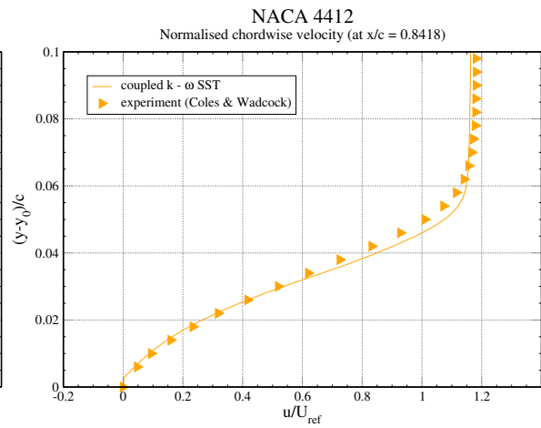
(d) x/c = 0.8418 ,
