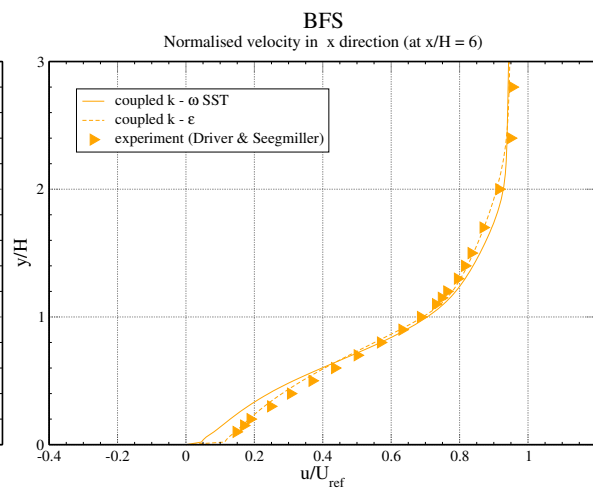
(d) x/H = 6 ,
