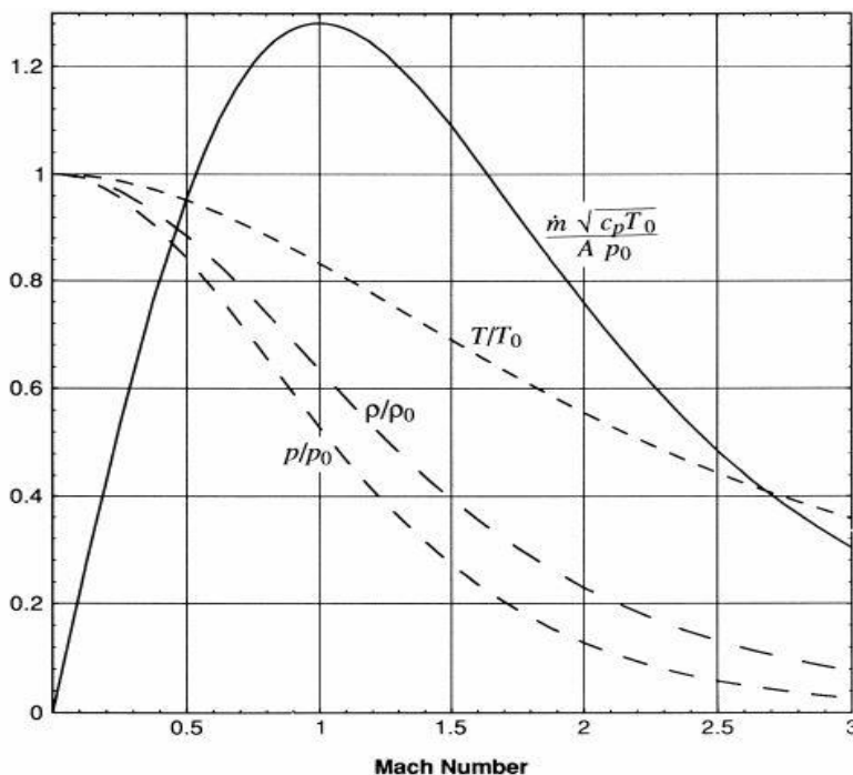
Slika 4: Ovisnost bezdimenzijskog masenog protoka o Machovom broju, [5]
