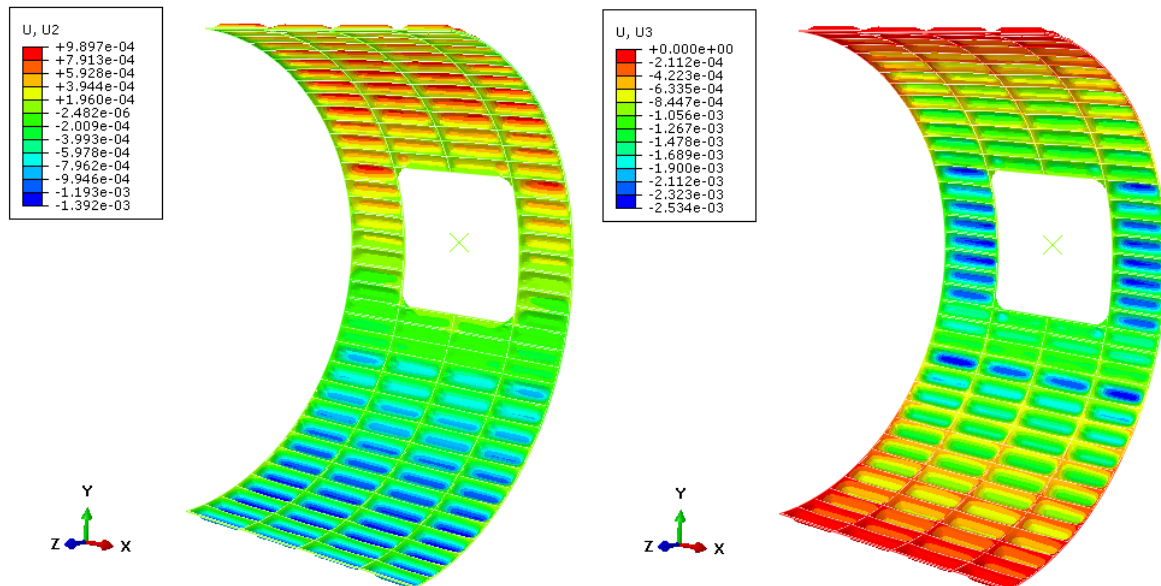
Slika 41. Raspodjela pomaka u smjeru osi y (lijevo) i pomaka u smjeru osi z (desno) [m]
