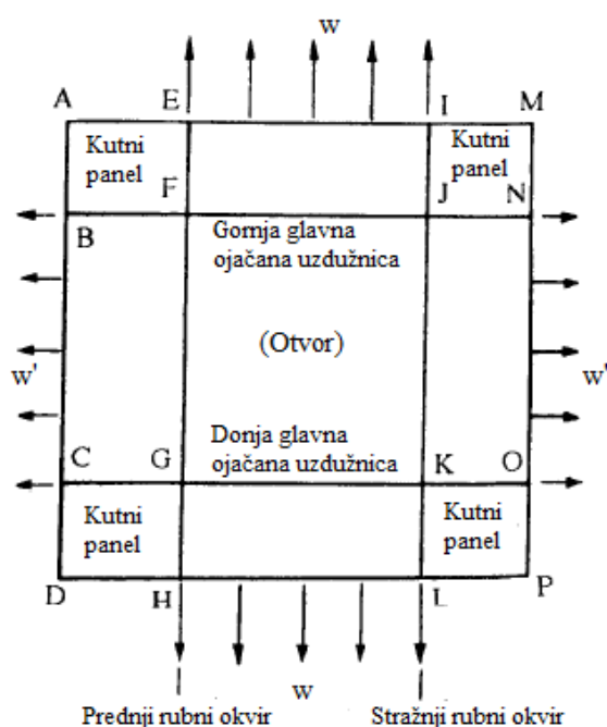
Slika 22. Raspored točkaka na panelima [3]
