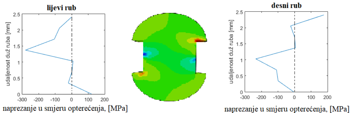
Slika 52. Raspodjela naprezanja u smjeru opterećenja po zakovici za model bez zračnosti, [MPa]
