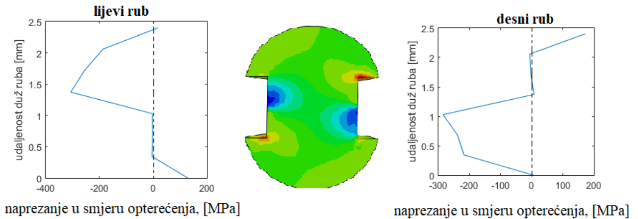
Slika 53. Raspodjela napreznja u smjeru opterećenja po zakovici za model sa zračnošću, [MPa]
