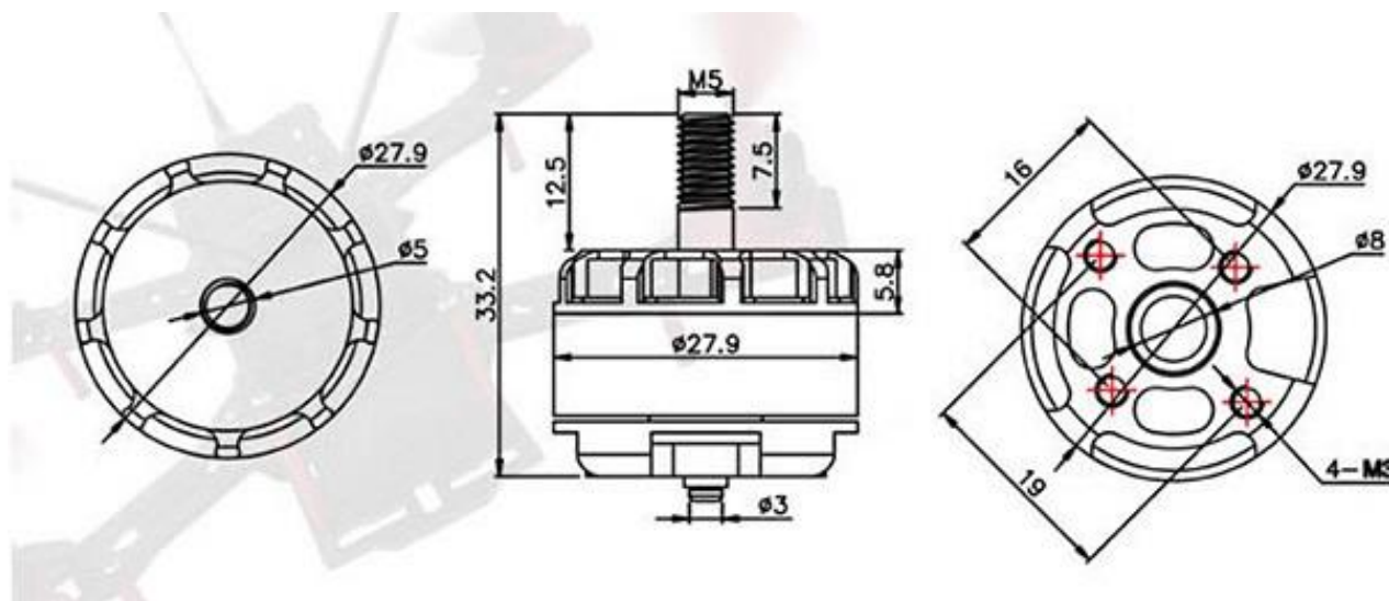
Slika 10. Dimenzije motora [20]
