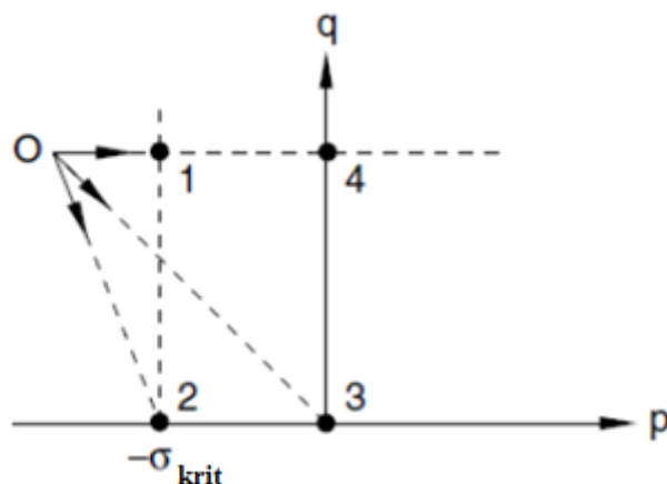
Slika 4 Prikaz promjene devijatorske ( q ) i hidrostatske ( p ) komponente ovisno o stanju napreznaja [9]
