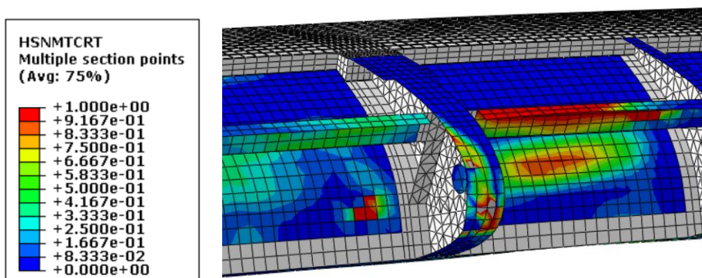
Slika 63 Vrijednosti indeksa Hashin-ovog kriterija popuštanja matrice pri vlačnom opterećenju - prikaz bez gornje oplata-CEL-110-GR-komp (t=0.00168 s)
