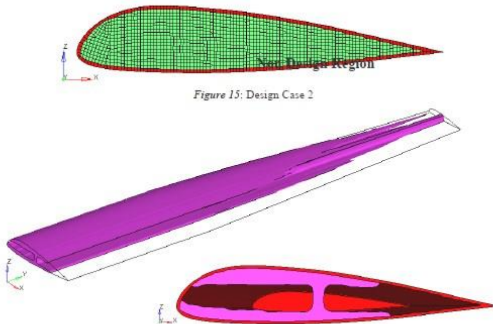
Slika 33 Topološki optimizirano krilo s jednom ramenjačom [14]
