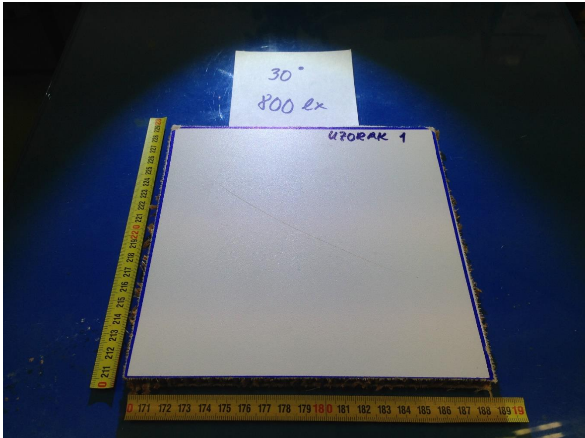
Slika 33 Fotografija provedenog ispitivanja Uzorka 1 pod upadnim kutom svjetlosti od 30° u odnosu na površinu ispitnog uzorka
