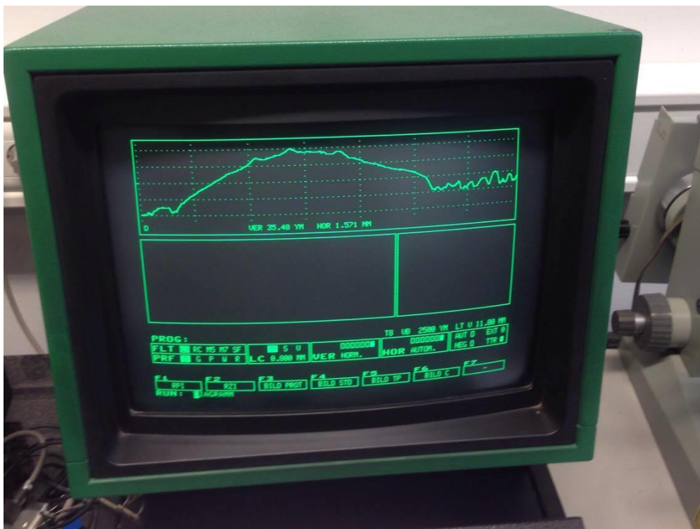
Slika 55 Prikaz snimljenog profila kapljice Uzorka 3 na računaru poveznim s ticalom za snimanje profila hrapavosti površine
