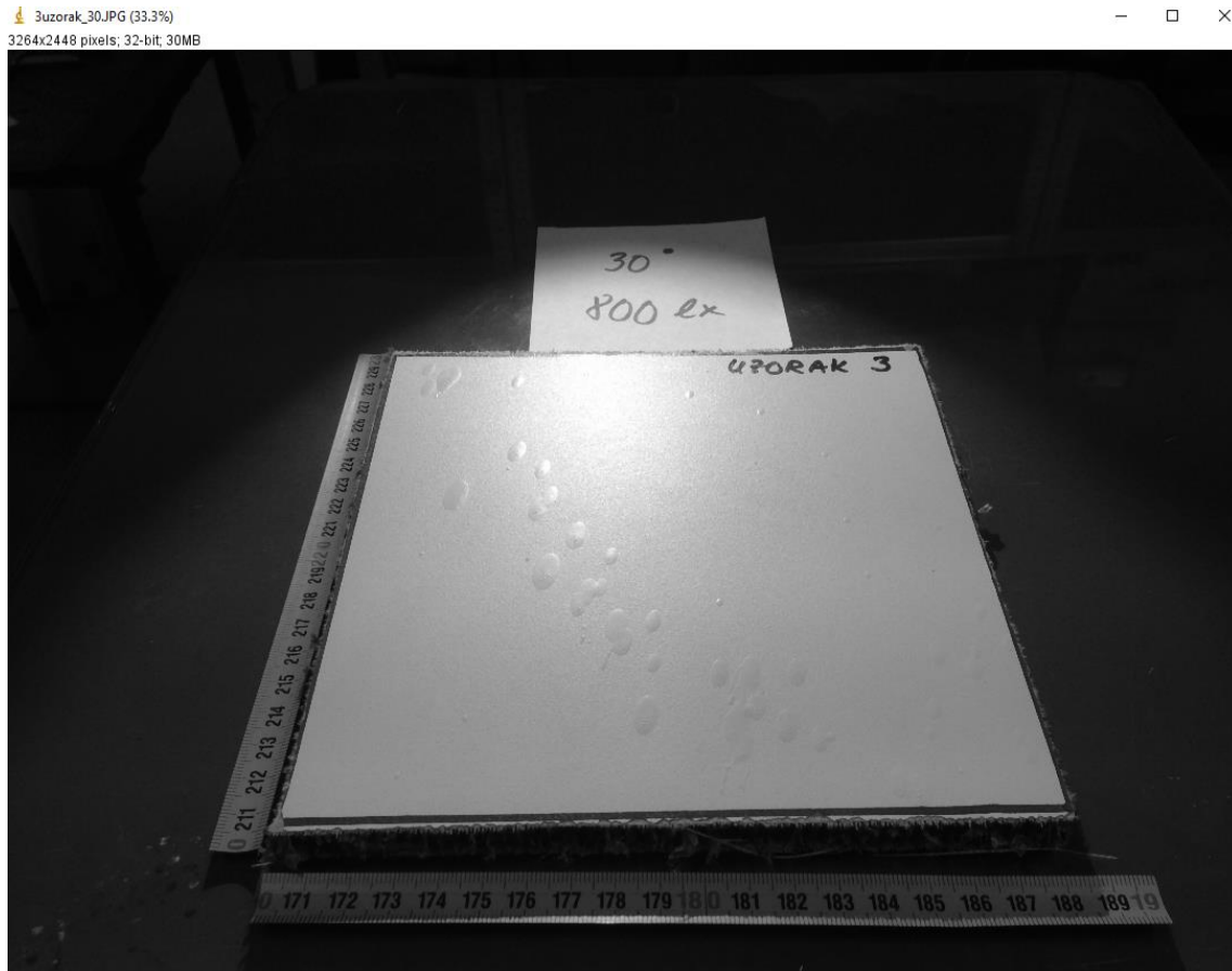
Slika 40 Uzorak 3 s upadnim kutom svjetlosti od 30^\circ u odnosu na površinu ispitnog uzorka, obrađen u ImageJ-u pomoću 32 bitnog greyscale transformatora i Median filtera
