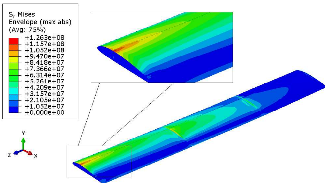
Slika 5.4 Ekvivalentno napreznje prema von Mises-u [Pa]
