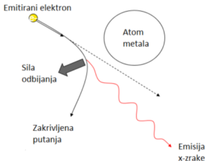
Slika 3.1: Zakočno zračenje [15]
