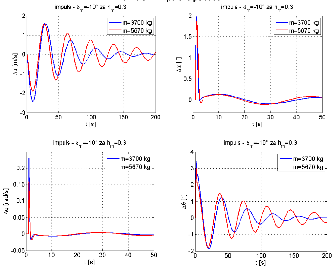
Slika 35. Odziv otvorenog sustava na impulsnu pobudu za LM1 i LM2
