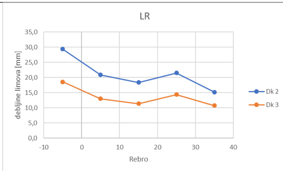
Slika 35. Promjena debljina limova po visinama prema LR-u
