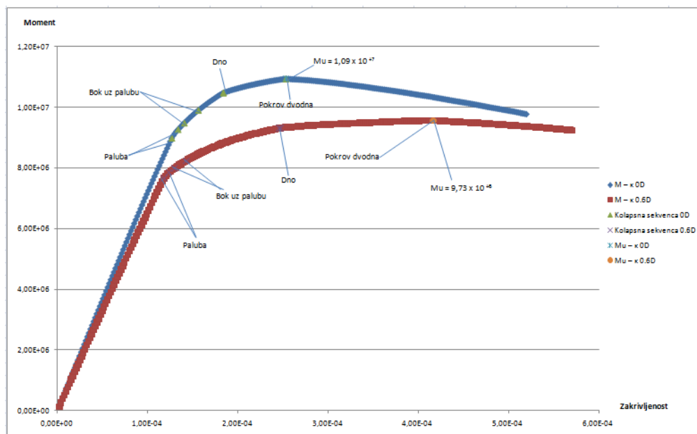
Slika 19. Kolapsna sekvenca za stanja 0D i 0.6D u slučaju pregiba (P3)
