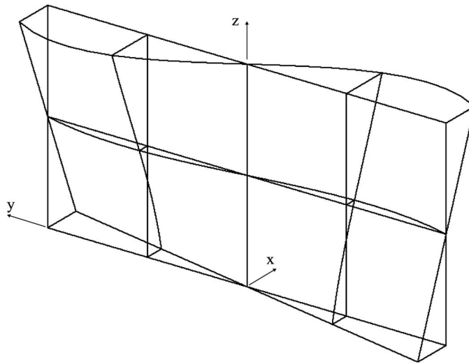
Slika 3.2.2.1 Deformacija pregrade [6]
