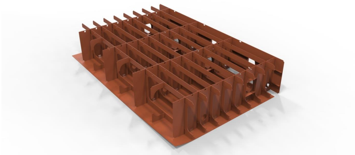
Slika 28. Sekcija dvodna bez pokrova
