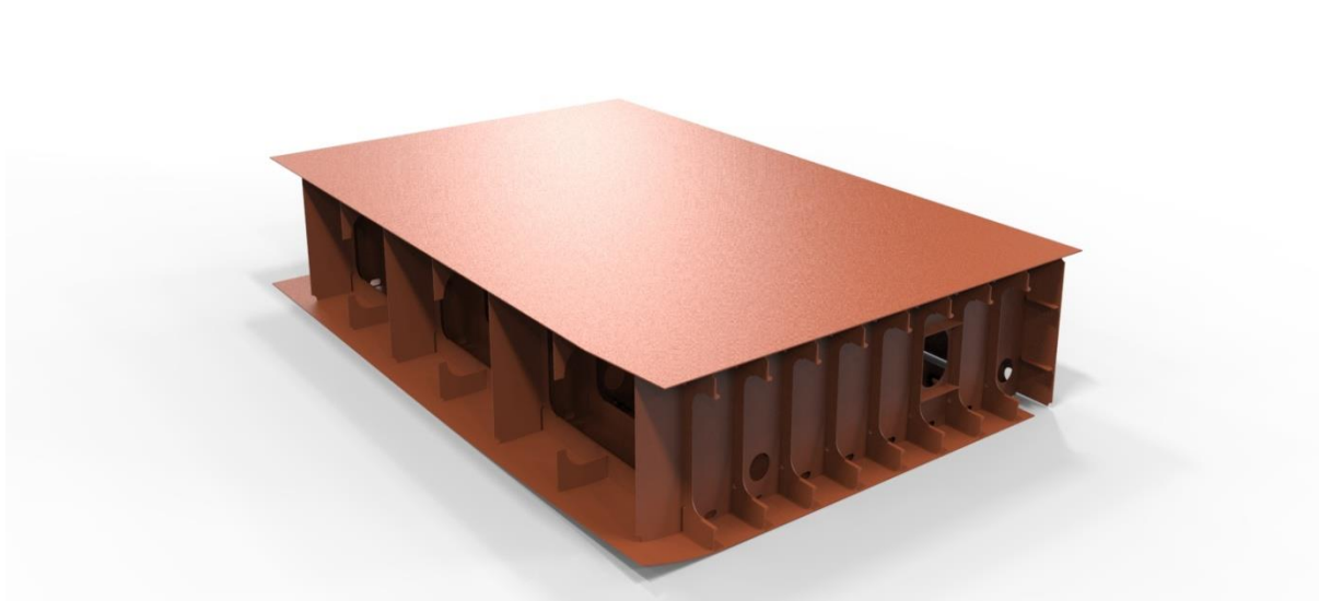
Slika 27. Sekcija dvodna
