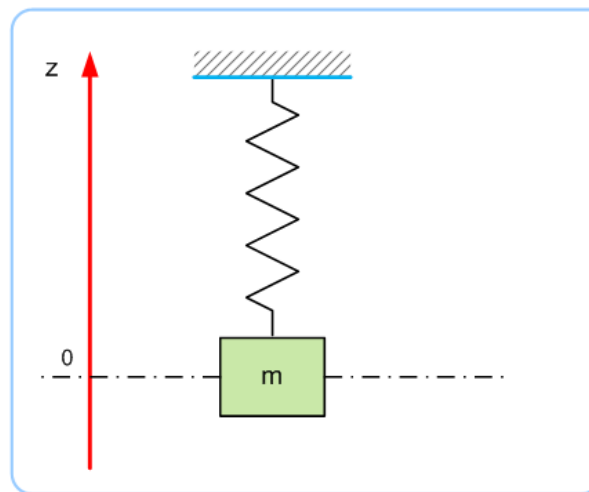
Slika 53 Uobičajeni prikaz harmoničkog oscilatora
