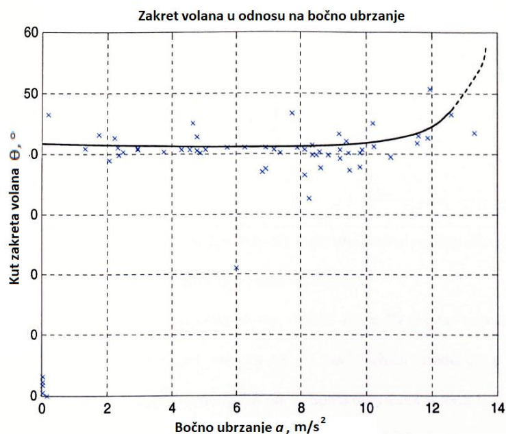
Slika 33. Mjerenja skretanja
