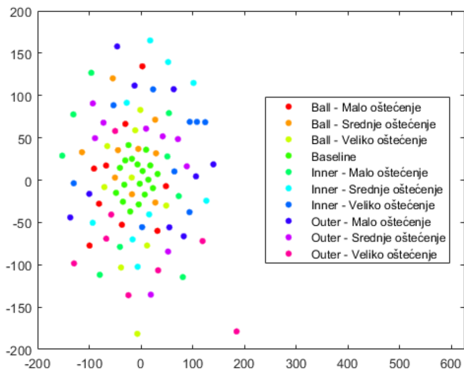
Slika 35. Vizualizacija značajki na ulaznom sloju konvolucijske neuronske mreže uz pomoć t-SNE algoritma
