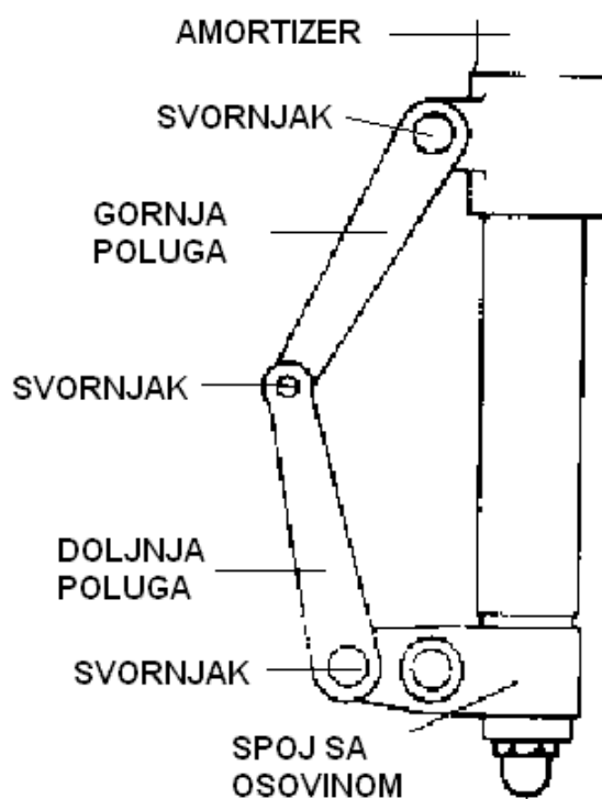
Slika 10: Antitorzijske poluge
