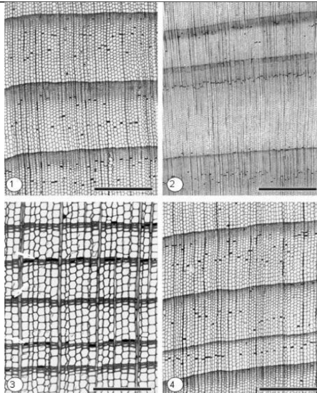
Slika 16. Aksijalni parenhim [15]
