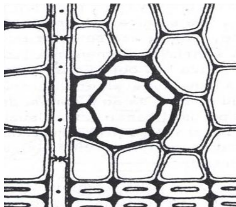
Slika 17. Smolenica [16]
