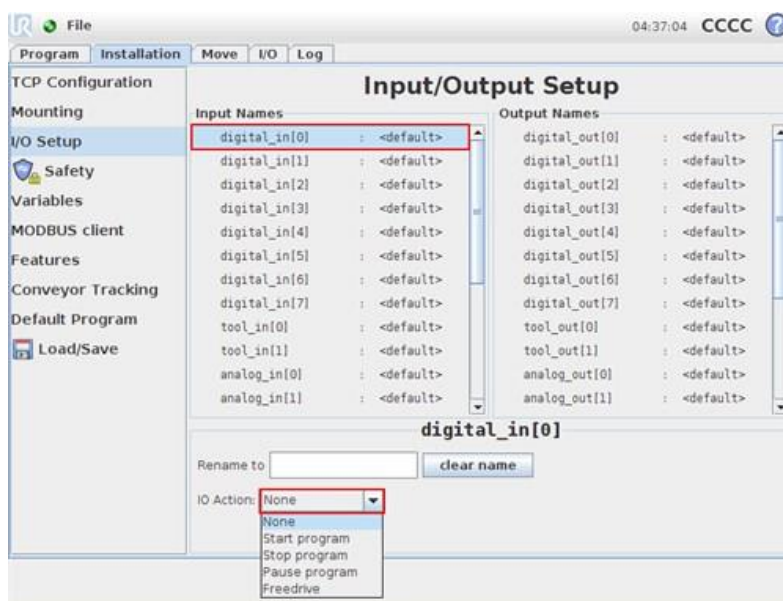
Slika 29. Dodjeljivanje posebnih uloga digitalnim ulazima [14]
