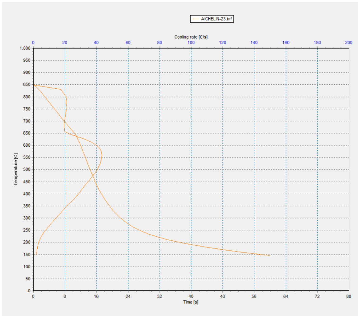
Slika 15. Karakteristike ohlađivanja ispitivanog uzorka ulja za kaljenje oznake AICHELIN-23°C
