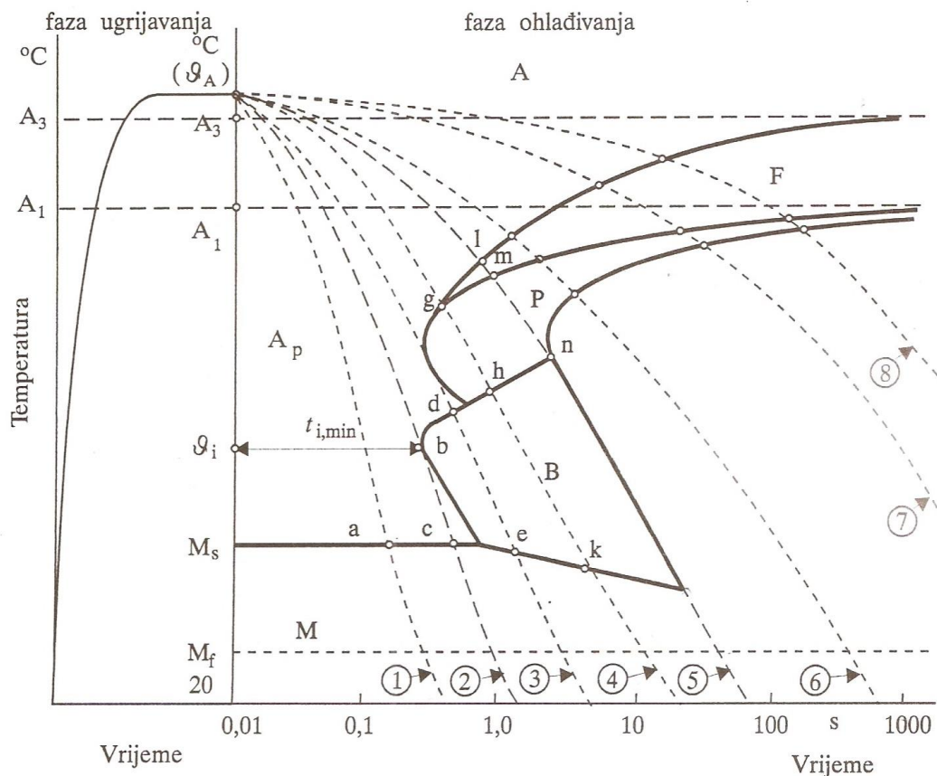
Slika 4. TTT dijagram kontinuiranog hlađenja jednog podeutektoidnog čelika [1]
