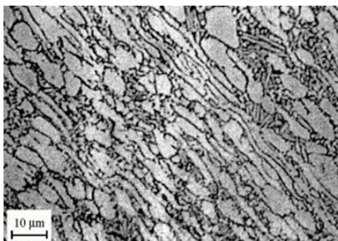
Slika 2.1 Mikrostrutura legure TiAl6V4 [4]
