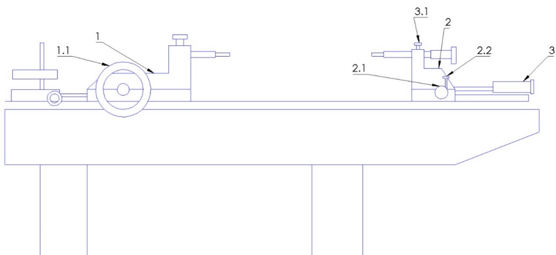
Slika 5- Shematska slika mjernog uređaja za mjerenje duljina do 3 metra
