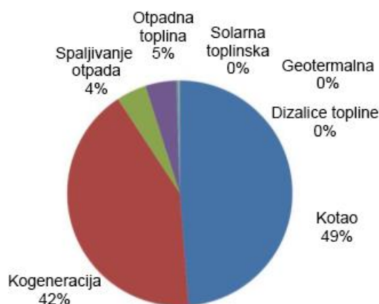
Slika 7. Postotak instalirane snage CTS prema tehnologiji [7]
