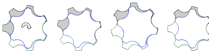
Slika 32. Varijacija površine istiskivanja [3]
