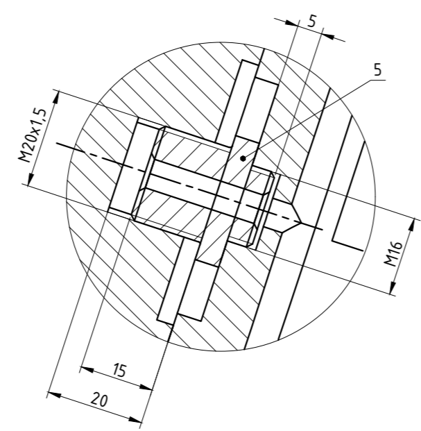
Detalj H M 1:1
