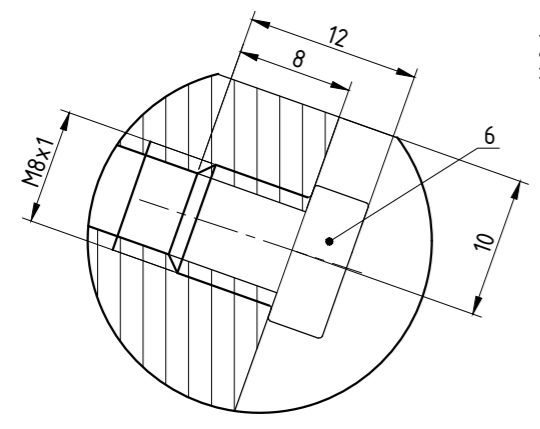
Detalj L M 2:1
