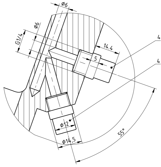
Detalj M M 1:1
