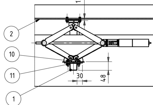
Presjek C-C M 1:10
