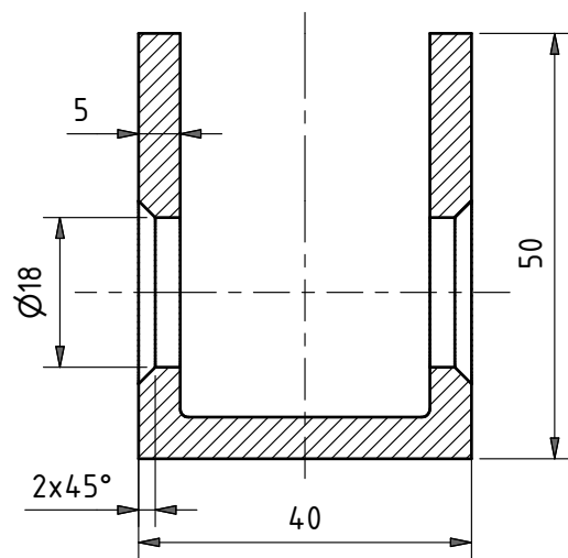
Presjek B-B
