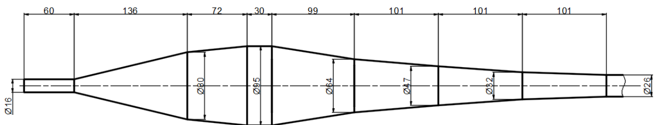
Slika 3.26. Rezonantni ispuh C
