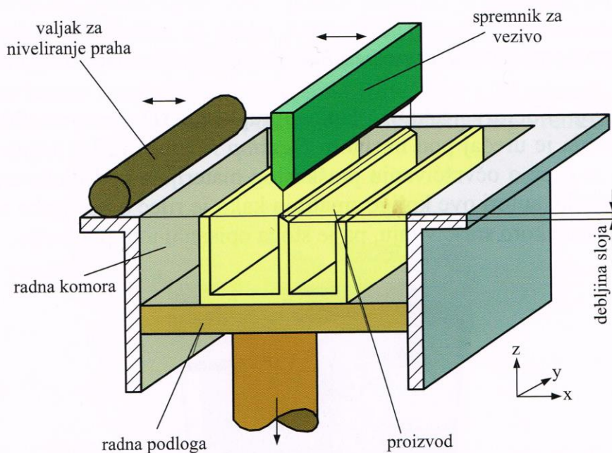
Slika 8. Načela rada postupka 3D tiskanja [1]
