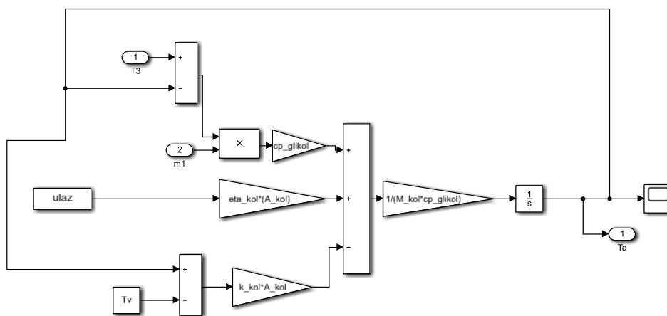
Schema 2 Segment kolektora
