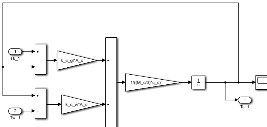
Shema 7 Segment cijevi toplinskog spremnika
