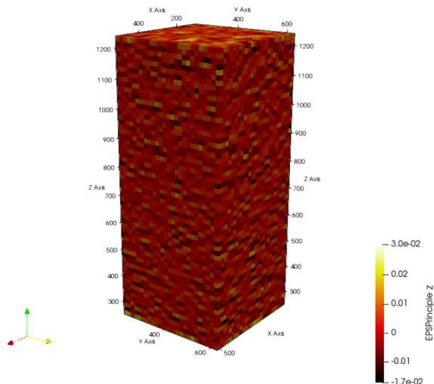
Slika 39. Polje deformacija u z smjeru za elemente veličine 16 voxela.
