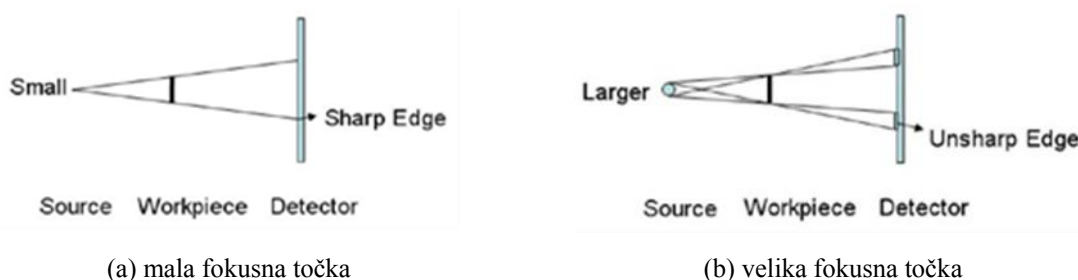
Slika 13. Efekt fokusne točke [1].
