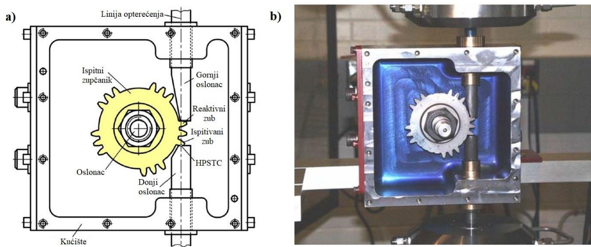
Slika 8. NASA-in ispitni uređaj: a) shema, prema [13] b) stvarni postav [12]
