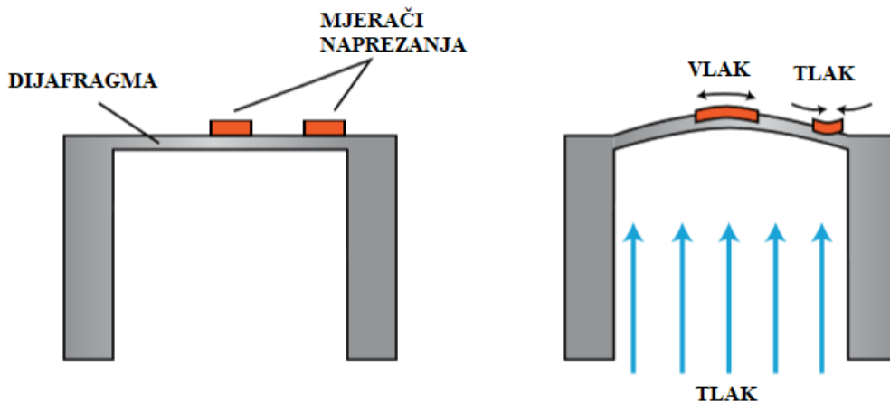
Slika 7. Otporni senzor
