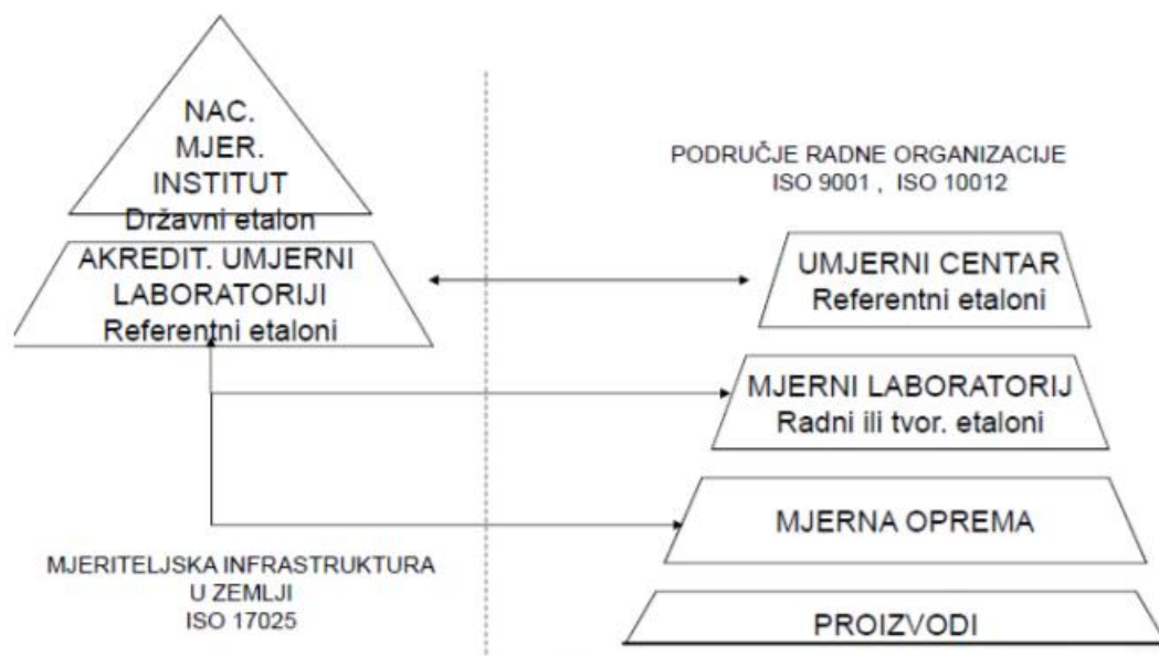
Slika 24. Shema umjeravanja.
