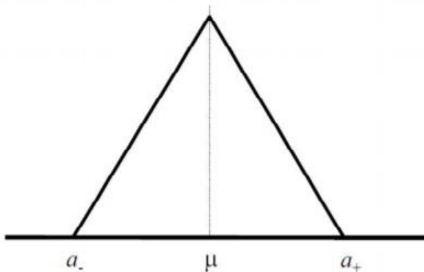
Slika 19. Trokutasta razdioba
