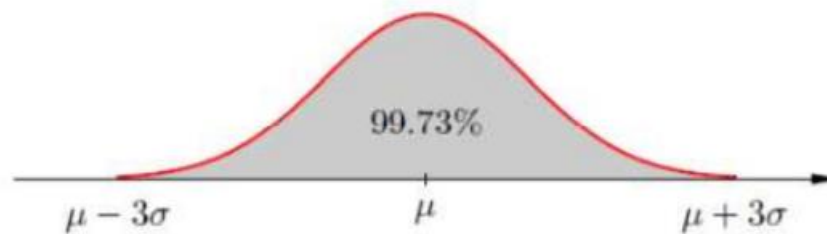
Slika 22. k=3
