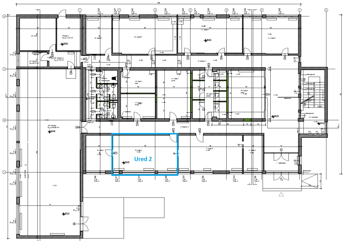
Slika 1: Tlocrt prizemlja uredske zgrade
