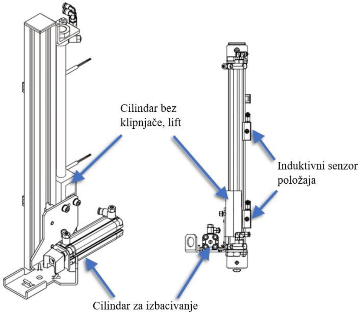
Slika 11. Modul lifta [4]
