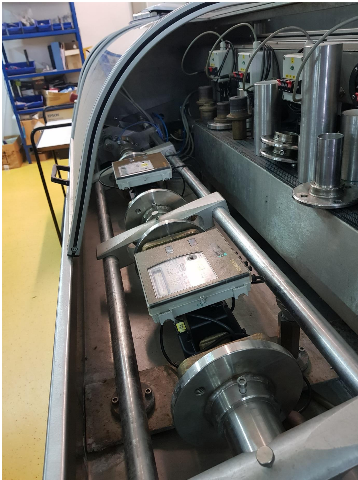
Slika 19. Mjerilo protoka spojeno na mjernu liniju
