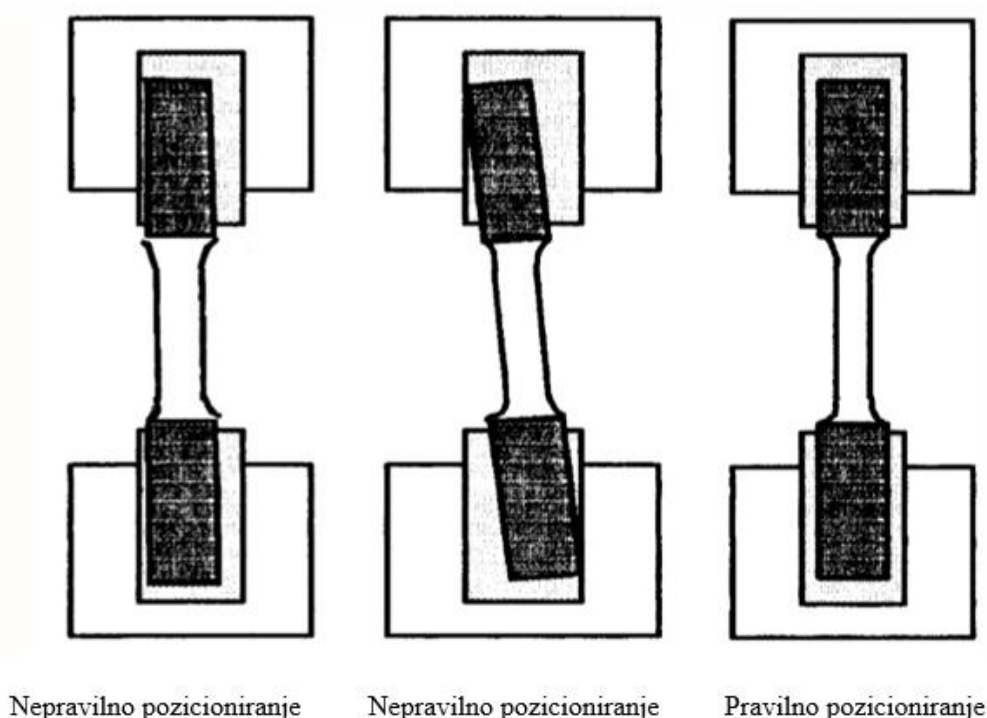
Slika 2.11. Neppravilno i pravilno pozicioniranje epruvete [2]
