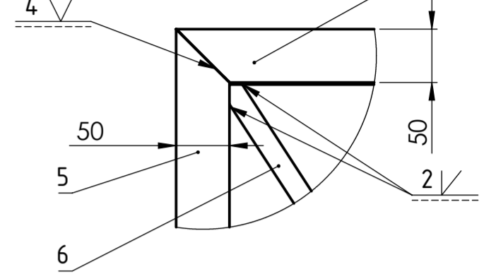
E (MJERILO 1 : 5)
