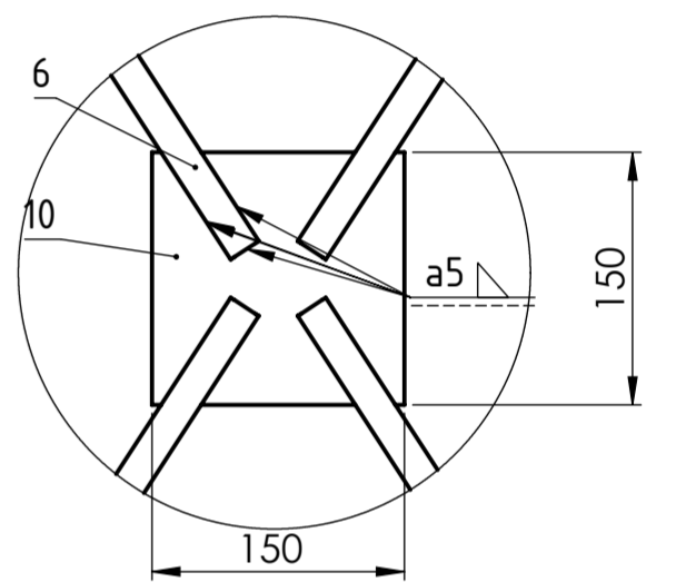
H (MJERILO 1 : 5)
