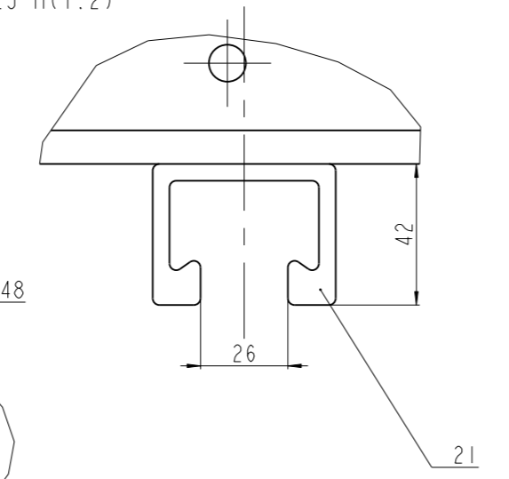
DETALJ H(1:2)
