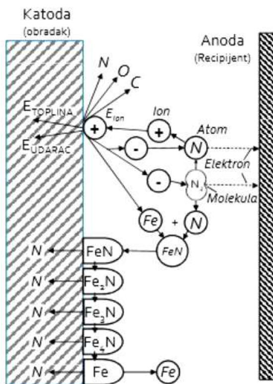
Slika 8. Koebel-ov model nitriranja u plazmi [11]
