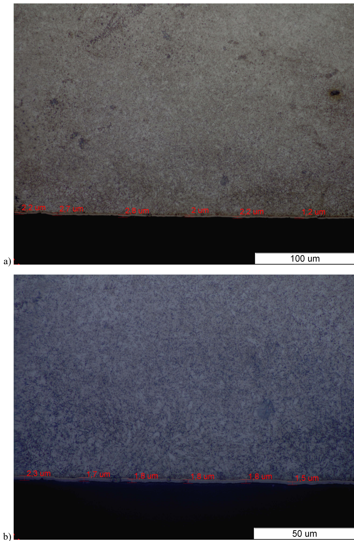
Slika 33. Površinski sloj na uzorku A2 : a) povećanje 500 puta, b) povećanje 1000 puta (nagriženo u 3%-tnom Nitalu)
