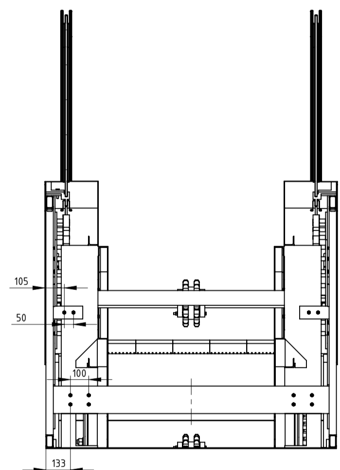
B-B (1:20)
