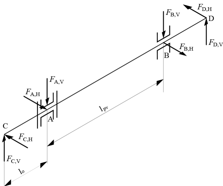
Slika 51. Opterećenje pune osovine
