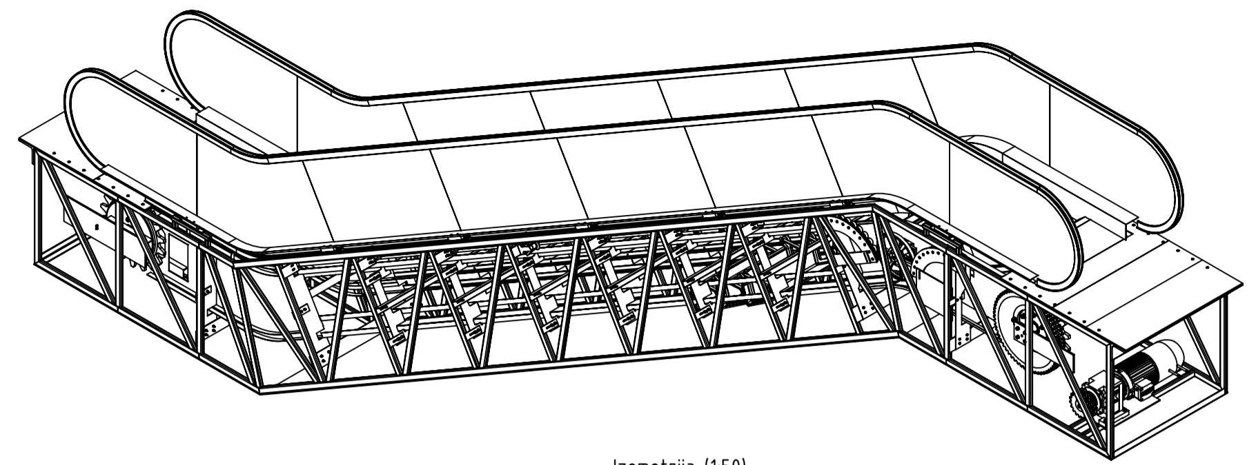
Izometrija (1:50)
