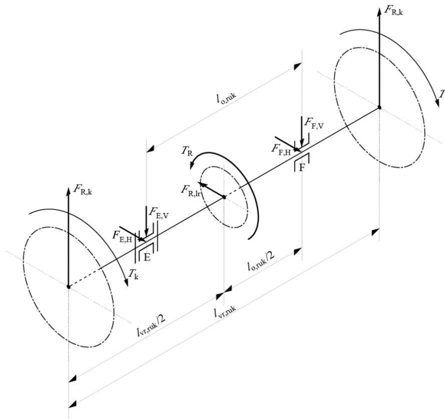
Slika 54. Opterećenje vratila rukohvata u izometriji
