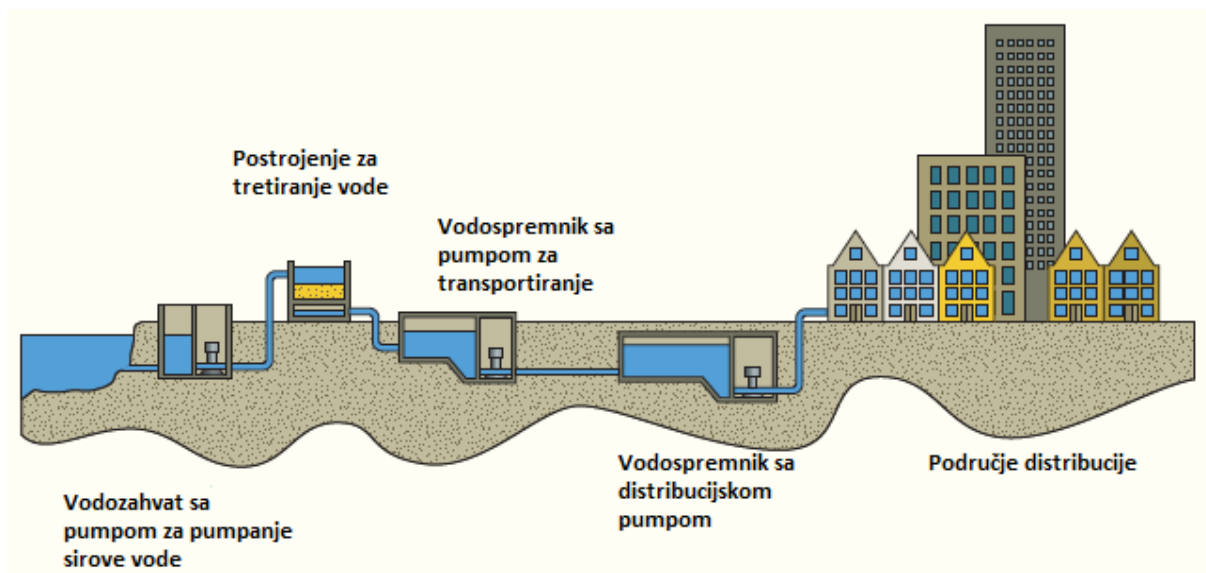
Slika 6. Pojednostavljena ilustracija izgleda vodoopskrbnog sustava [9]
