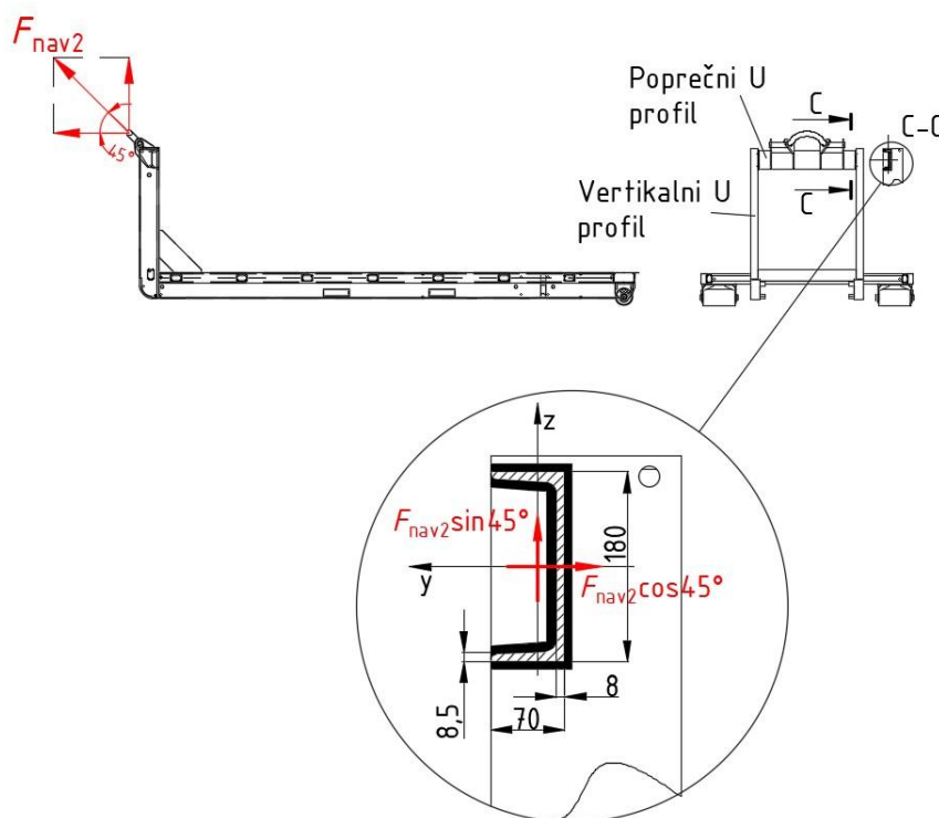
Slika 3.66. Shema opterećenja i presjek zavara poprečnog U profila
